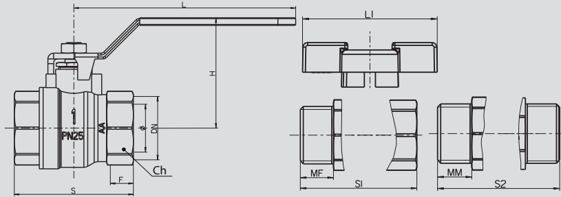
DIMENSÕES - (mm)
