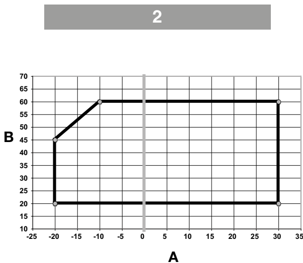
Diagrama caudal-carga hidrostática
